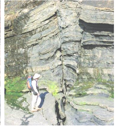
الوثيقة 1 صور للتشوهات طبقات القشرة الأرضية
