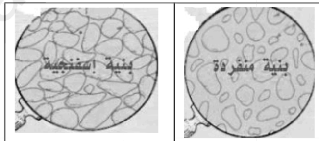
السند 01: رسم تخطيطي يوضح بنية التربة في المنطقتين
